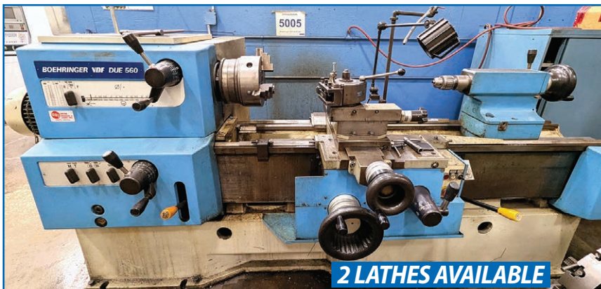
2 LATHES AVAILABLE BOEHRINGER VDF DUE 560 LATHE
