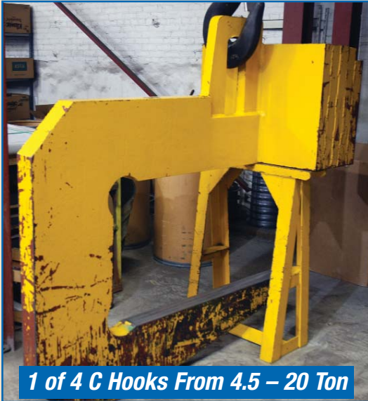
20 TON C HOOK
